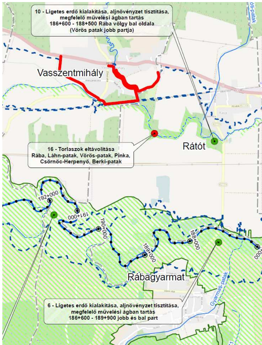
Intézkedési javaslat (Rába nagyvízi mederkezelési terv)
